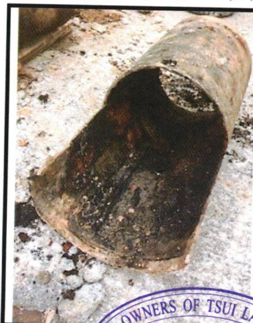
←2019 年 9 月翠麗迴旋處掘出消防喉內部生銹狀況
